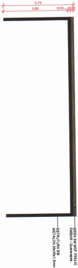
2 CORTE AA ESCALA 1 : 15
