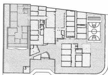
Planta Baixa Edificações
