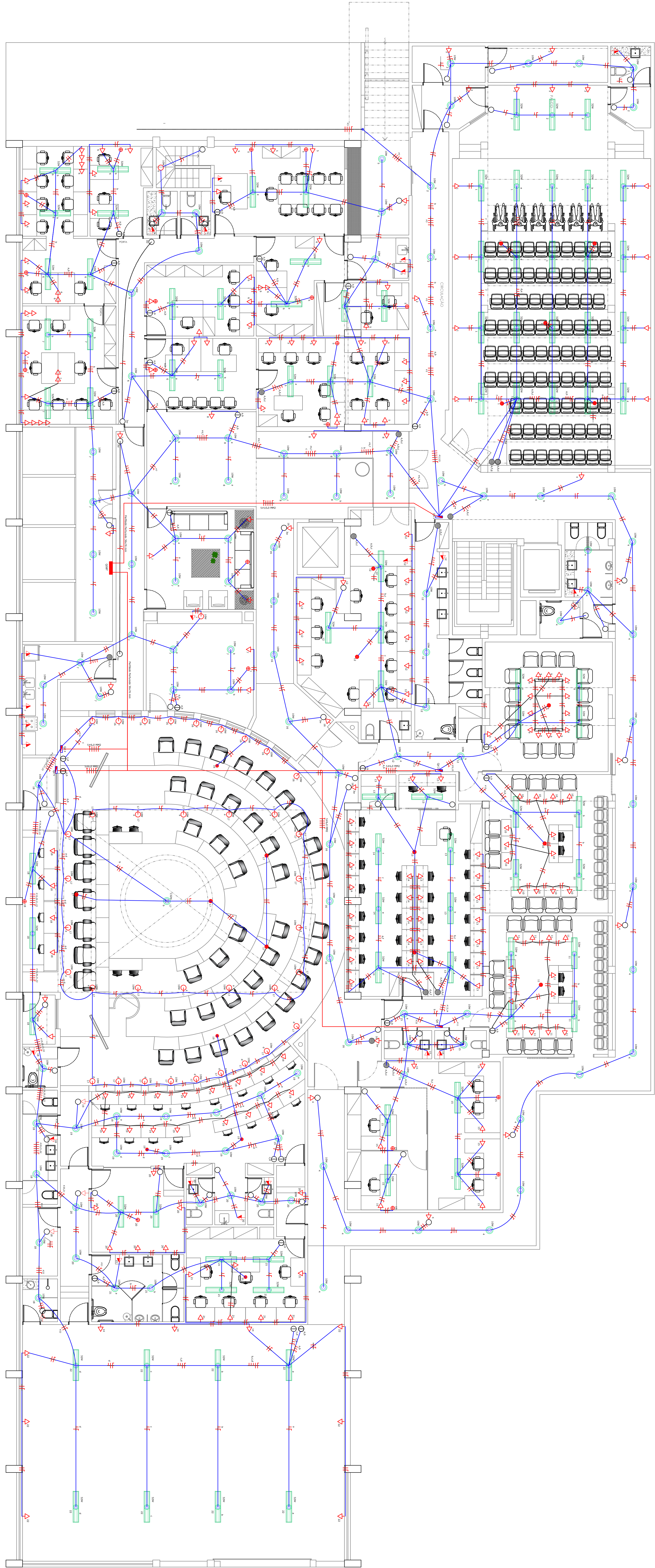
PLANTA BAIXA - SEMI-ENTERRADO CIRCUITOS DE LUZ E FORÇA ESCALA: 1/25
